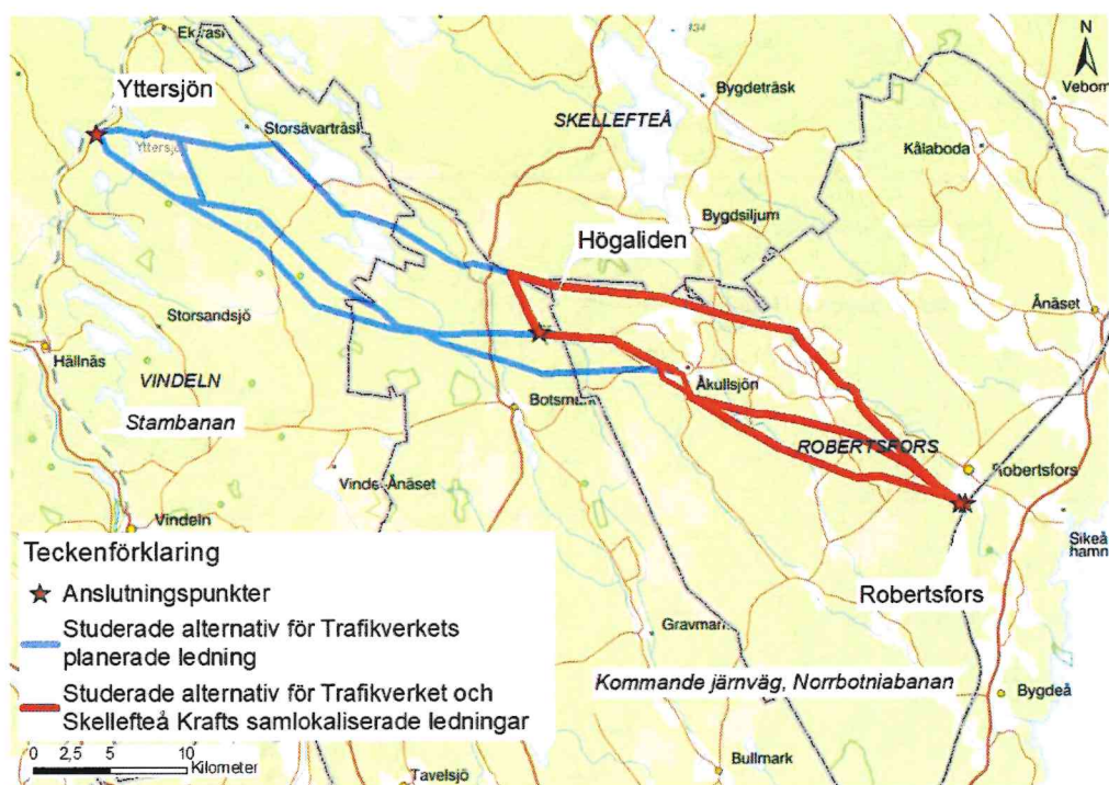
Figur 1-2, Trafikverket och Skellefteå Krafts studerade stråkalterantiv.
