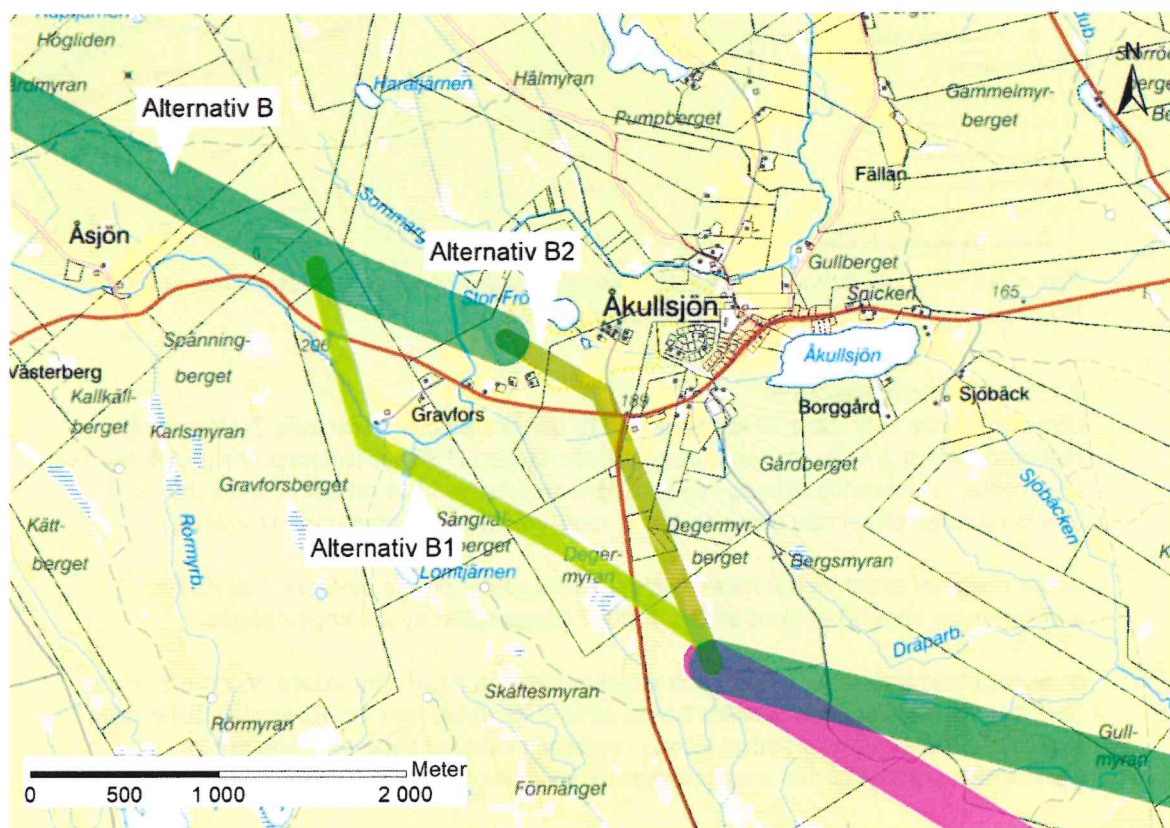
Figur 2-2. Alternativ B1 och B2 vid Åkullsjön.
